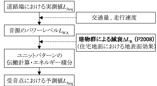
図-10 建物背後の騒音レベルを求める手順
