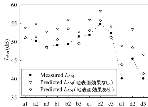
図-11 予測値と実測結果の比較
