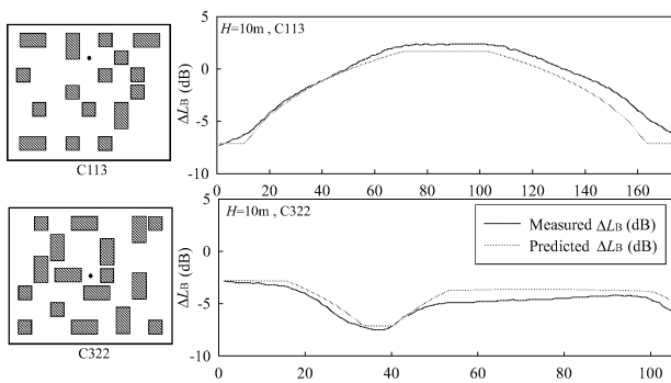
図-6 騒音減衰量 \Delta L_B のユニットパターンの比較
